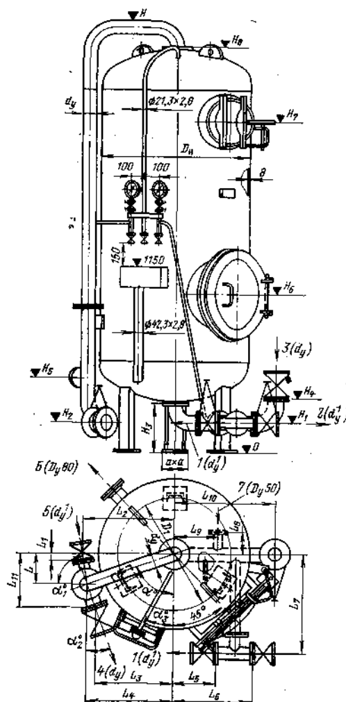
Рис. 7-1. Фильтры осветлительные диаметром 1000 и 1500 мм (БиКЗ), см. табл. 7-2. 1 — выход обработанной воды; 2 — спуск первого фильтрата; 3 — подвод промывочной воды; 4 — спуск промывочной воды; 5 — подвод обрабатываемой воды; 6 — штуцер D_y = 80 мм для гидровыгрузки, установлен на отметке у фильтра диаметром: 1000—580 мм, 1500—745 мм; 7 — подвод сжатого воздуха.
