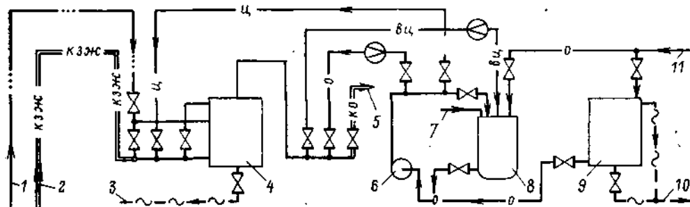
Рис. 2-17. Схема обезжелезивания конденсата в целлюлозных фильтрах намывного типа. 1 — сжатый воздух; 2 — зажелезенный конденсат; 3 — сброс целлюлозы в водоотвал; 4 — целлюлозный намывной фильтр; 5 — обезжележенный конденсат; 6 — насос для намыва целлюлозы; 7 — загрузка целлюлозы; 8 — гидроразбиватель целлюлозы; 9 — бак осветленной воды; 10 — дренаж; 11 — осветленная вода.
