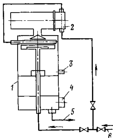
Рис. 13-8. Схема компоновки вертикального вакуумного деаэратора с поверхностным охладителем выпара.
