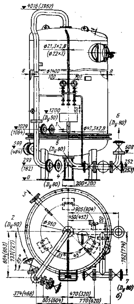
Рис. 7-15. Фильтры натрий- и водород-катионитные первой ступени (нижнее рас- предустройство — ложное дно выполнено из пресс-материала АГ-4с). БИКЗ.
