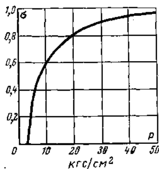
Рис. 4-1. Зависимость разложения Na_2CO_3 от давления в котле.
