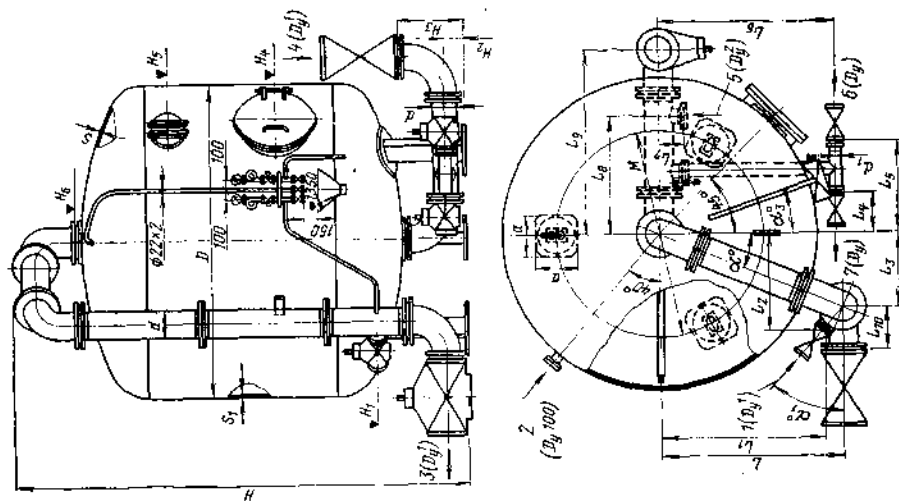
Рис. 7-3. Фильтры осветительные диаметром от 2000 до 3400 мм (МКЗ), см. табл. 7-3.
