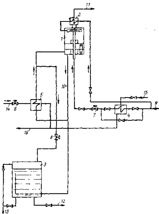
Рис. 13-14. Принципиальная схема деаэрационно-подпиточной установки без потерь конденсата с естественной циркуляцией греющей среды.
