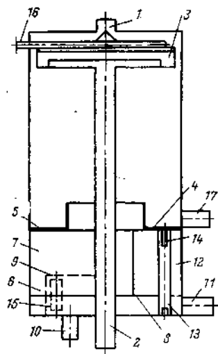
Рис. 13-6. Принципиальная схема вакуумного барботажного деаэратора.
