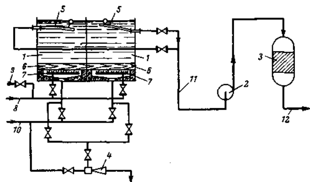
Рис. 6-3. Схема склада мокрого хранения коагулянта. 1 — железобетонный бак мокрого хранения коагулянта; 2 — насос раствора коагулянта; 3 — фильтр раствора коагулянта; 4 — водоводяной насос для удаления грязи из резервуара; 5 — гибкий плавающий шланг для отвода отстоявшегося крепкого раствора коагулянта; 6 — деревянные доски, поставленные на ребро; 7 — перфорированный трубопровод для барботажного воздуха; 8 — подвод сжатого воздуха; 9 — подвод пара; 10 — подвод воды для растворения коагулянта и к водоводяному насосу; 11 — крепкий раствор коагулянта; 12 — осветленный раствор коагулянта к расходному баку.
