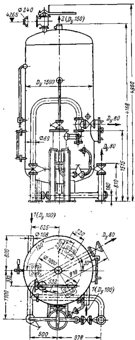
Рис. 7-42. Расширитель непрерывной продувки первой ступени СП-5,5 (ТКЗ). 1 — вход продувочной воды; 2 — выход отсепарированного пара.
