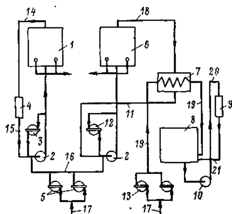
Рис. 2-2. Схема магнитной обработки воды в котельной с водогрейными чугунными секционными котлами (для артезианской воды с J_K \leq 9 мг-экв/л; содержанием кислорода не более 3 мг/л и подогревом воды до t < 95^\circ C ).
