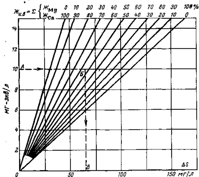
Рис. 4-2. Увеличение сухого остатка воды ( \Delta S ) при ее обработке по схеме натрий-катионирования в зависимости от жесткости исходной воды ( J_{н,в} ).
