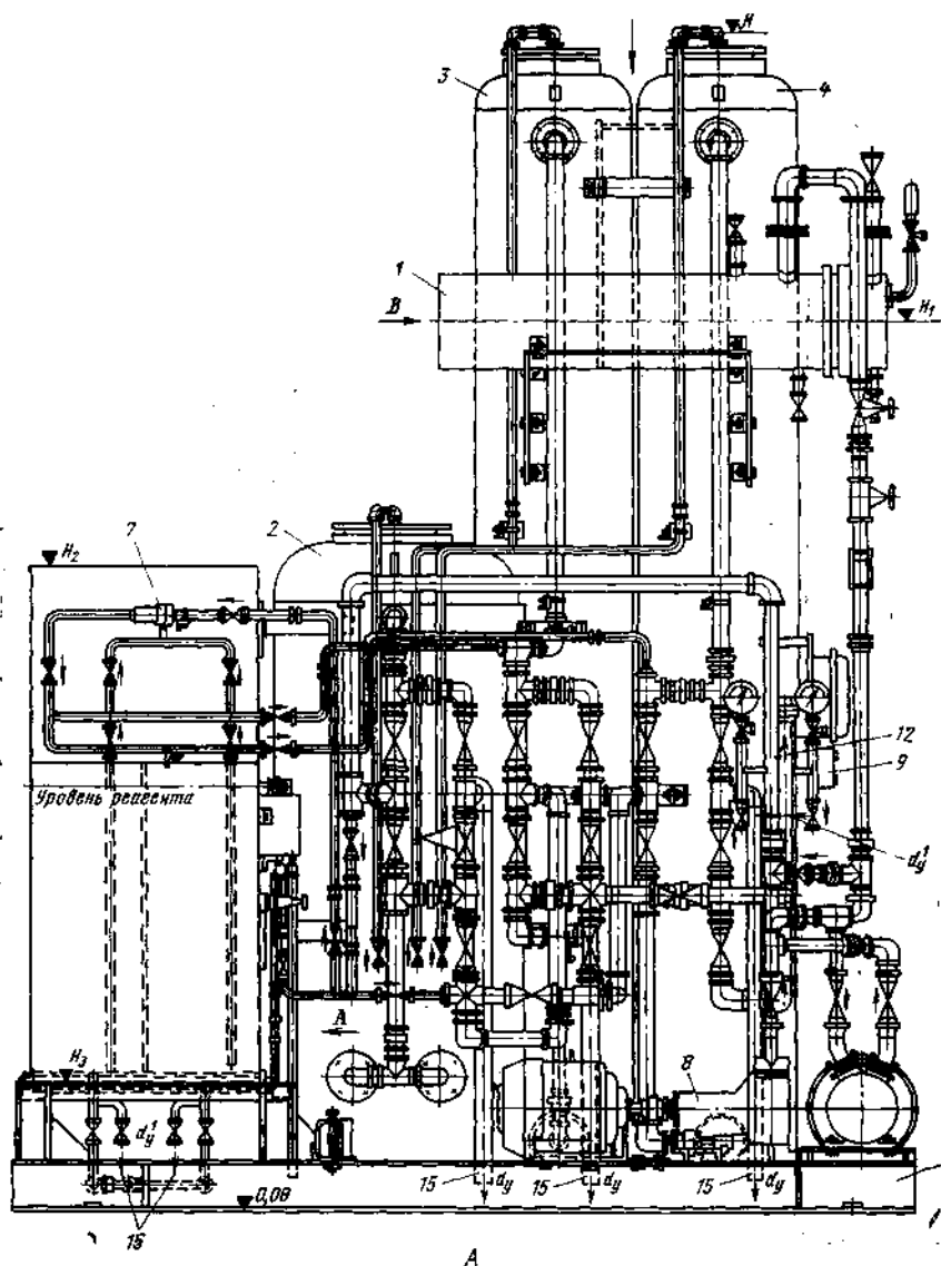
Рис. 7-47: Компонировка блочных водоподготовительных установок производительностью 5 и 10 м 3 /ч (СЗТМ), см. табл. 7-24.
