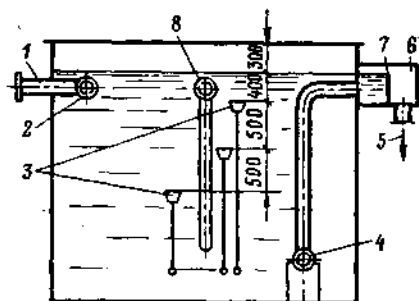
Рис. 2-16. Бак-отстойник конденсата.
