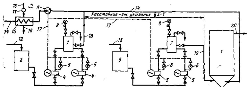
Рис. 6-7. Схема коагуляции в осветлителе с дозировкой полиакриламида (ПАА).
