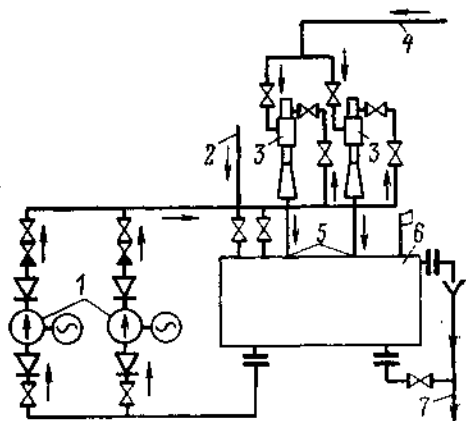
Рис. 13-10. Замкнутая схема включения водоструйных эжекторов.
