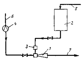
Рис. 6-10. Схема приготовления регенерационного раствора.
