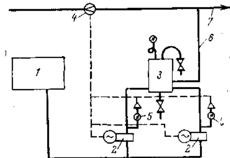
Рис. 2-12. Схема дозирования реагентов. 1 — бак раствора реагента; 2 — насос-дозатор типа НД; 3 — воздушный колпак; 4 — расходомерная шайба; 5 — электроконтактный манометр; 6 — дозируемый раствор реагента; 7 — химически очищенная или питательная вода.
