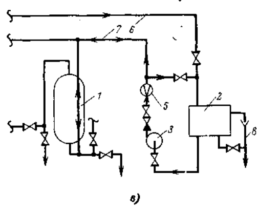
Рис. 6-9. Схема взрыхляющей промывки фильтров.
