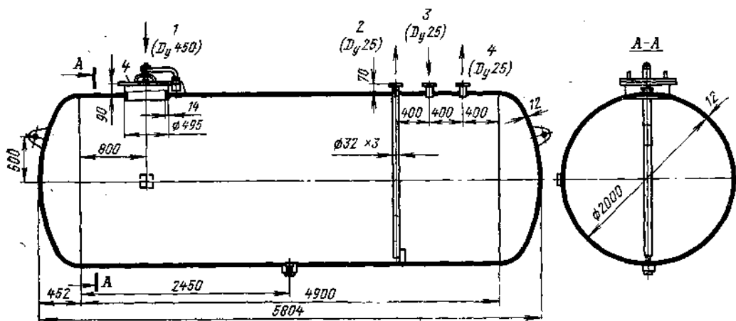
Рис. 7-32. Бак хранения крепкой серной кислоты емкостью 15 м³ (ТКЗ).
