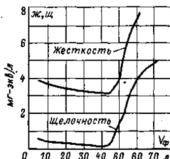
Рис. 2-6. График изменения жесткости ( Ж ) и щелочности ( Щ ) в процессе водород-катионирования с «голодной» регенерацией фильтров в зависимости от объема фильтрата ( V_{\phi} ). Качественные показатели исходной воды:
