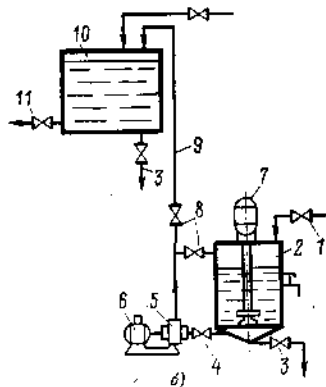
Рис. 8-8. Установка для приготовления растворов ПАА типа УРП-2М.
