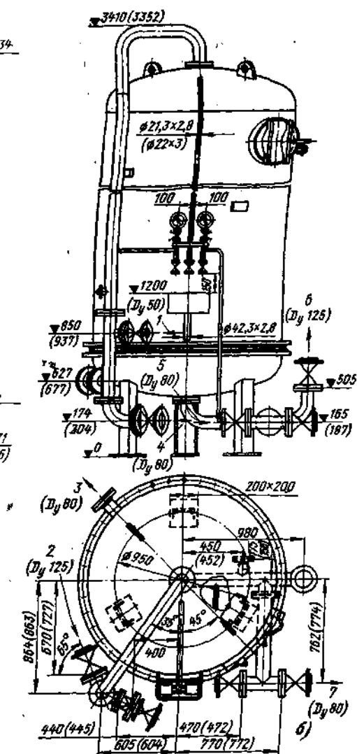
Рис. 7-16. Фильтры натрий- и водород-катионитные второй ступени (нижнее распределительное устройство — ложное дно выполнено из пресс-материала АГ-4с), БИКЗ.
