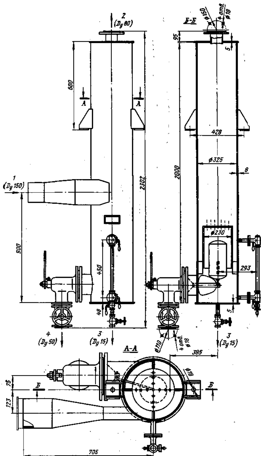
Рис. 7-39. Сепаратор непрерывной продувки D_y = 300 мм (с плоским дном), БикЗ. 1 — подвод продувочной воды; 2 — выход пара; 3 — спуск; 4 — выход отсепарированной воды.
