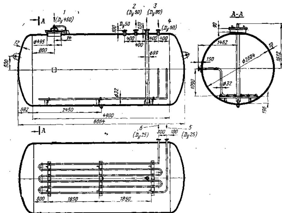
Рис. 7-33. Бак хранения едкого натра емкостью 30 м³ (ТКЗ).
