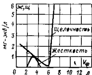
Рис. 2-8. График изменения щелочности и жесткости фильтрата (Щ, Ж) в процессе водород-катионирования с «голодной» регенерацией фильтров в зависимости от объема фильтрата ($V_{\phi}$). Качество исходной воды:
