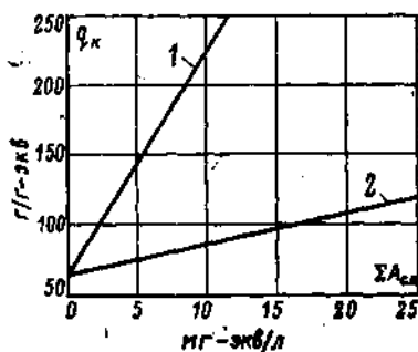
Рис. 5-6. Определение удельного расхода серной кислоты q_k на регенерацию водород-катионитных фильтров первой ступени в зависимости от суммарного содержания анионов сильных кислот \Sigma A_{\text{с.к.}} ( \text{SO}_4^{2-} и \text{Cl}^- ).
