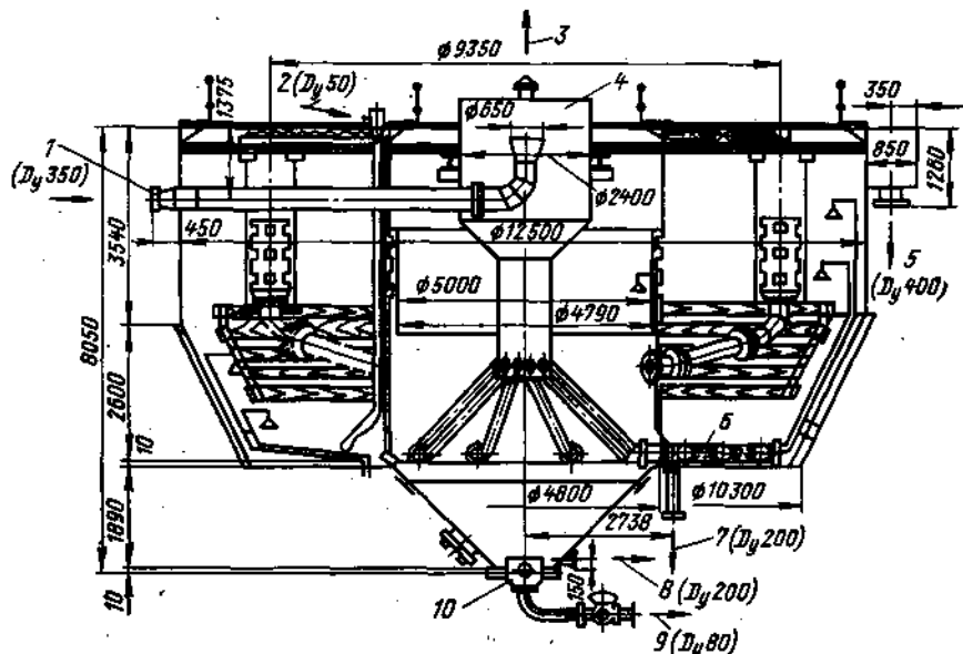
Рис. 8-6 Осветлитель для коагуляции воды типа ЦНИИ-3 (автор Е. Ф. Кургаев) произв. водительностью 450 м 3 /ч.
