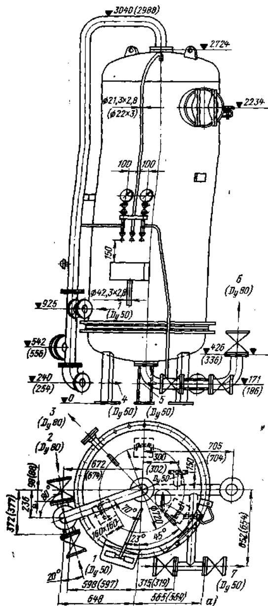
Рис. 7-16. Фильтры натрий- и водород-катионитные второй ступени (нижнее распределительное устройство — ложное дно выполнено из пресс-материала АГ-4с), БИКЗ.
