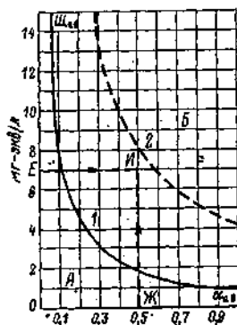
Рис. 4-3. Определение возможности применения схемы натрий-катионирования по концентрации уголекислоты в паре (при барботажной деаэрации).
