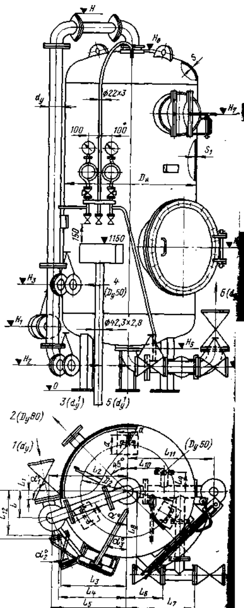
Рис. 7-14. Фильтры водород-катионитные второй ступени диаметром 1000 и 1500 мм (БикЗ), см. табл. 7-9.
