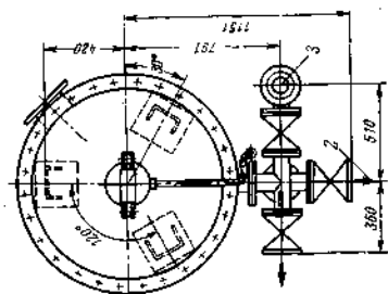
Рис. 7-58. Содержатель реактивов D_y = 1000 мм (СЗТМ). 1 — вход воды для растворения соли; 2 — вход промывочной воды; 3 — выход раствора соли; 4 — дренаж; 5 — фильтрующий материал; 6 и 7 — подводящие шланги.
