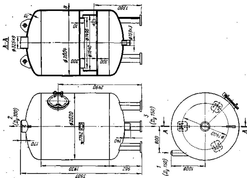
Рис. 7-44. Расширитель периодической продувки СП-7.5 (ТКЗ).
