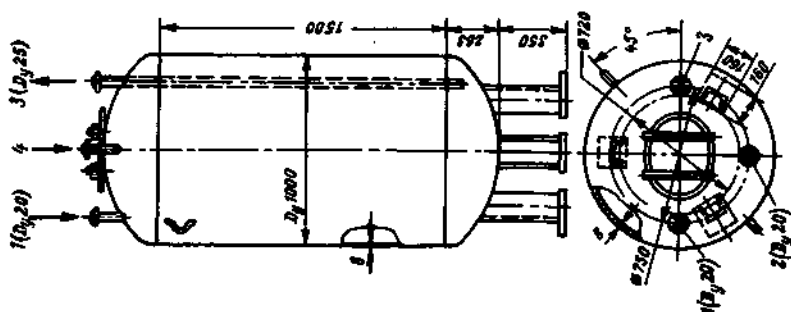
Рис. 7-31. Бак-вытеснитель крепкой серной кислоты емкостью 1,5 м 3 (БикЗ). 1 — подвод сжатого воздуха; 2 — воздушник; 3 — выход кислот; 4 — овальный люк для заливки кислоты.
