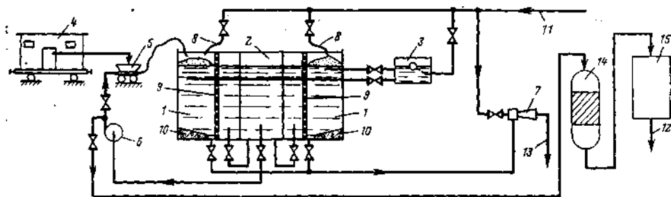
Рис. 6-2. Схема мокрого хранения соли с насосом крепкого раствора.
