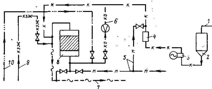
Рис. 2-18. Схема обезжелезивания конденсата на водород-катионитных фильтрах, загруженных сульфоглемом.
