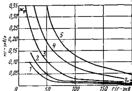
Рис. 5-5. Определение удельного расхода серной кислоты q_k в зависимости от требуемой жесткости фильтра Ж_f и общего соледержания исходной воды.
