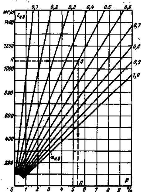
Рис. 4-6. Определение величины продувки котлов, %, в зависимости от сухого остатка обработанной воды S_{д.в} при S_{к.в} = 10\,000 мг/л.
