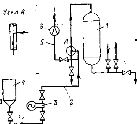
Рис. 6-11. Схема регенерации фильтра насосом-дозатором типа НД.
