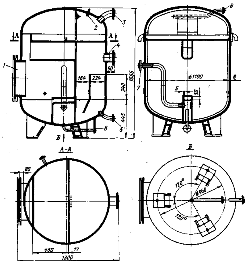
Рис. 13-2. Деаэратор типа ДСА-1.
