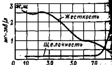
Рис. 2-7. График изменения жесткости ( Ж ) и щелочности ( Щ ) в процессе водород-катионирования с «голодной» регенерацией фильтров в зависимости от объема фильтрата ( V_{\phi} ). Качество исходной воды: Ж_0 = 8 мг-экв/л; Щ_{н.в} = 7,2 мг-экв/л; K = 0 ; A = 2,6 .
