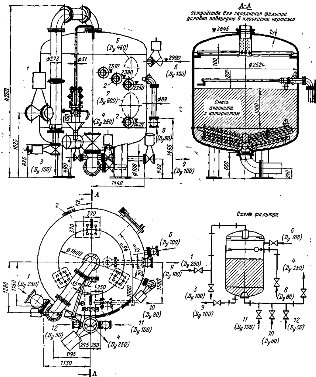
Рис. 7-22. Фильтр смешанного действия (ФСД) диаметром 2600 мм с выносной регенерацией (ТКЗ).
