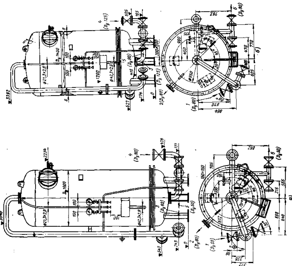
Рис. 7-2. Фильтры осветительные (нижнее распределительное — ложное, дно из пресс-материала АГ-4С), БМКЗ.
