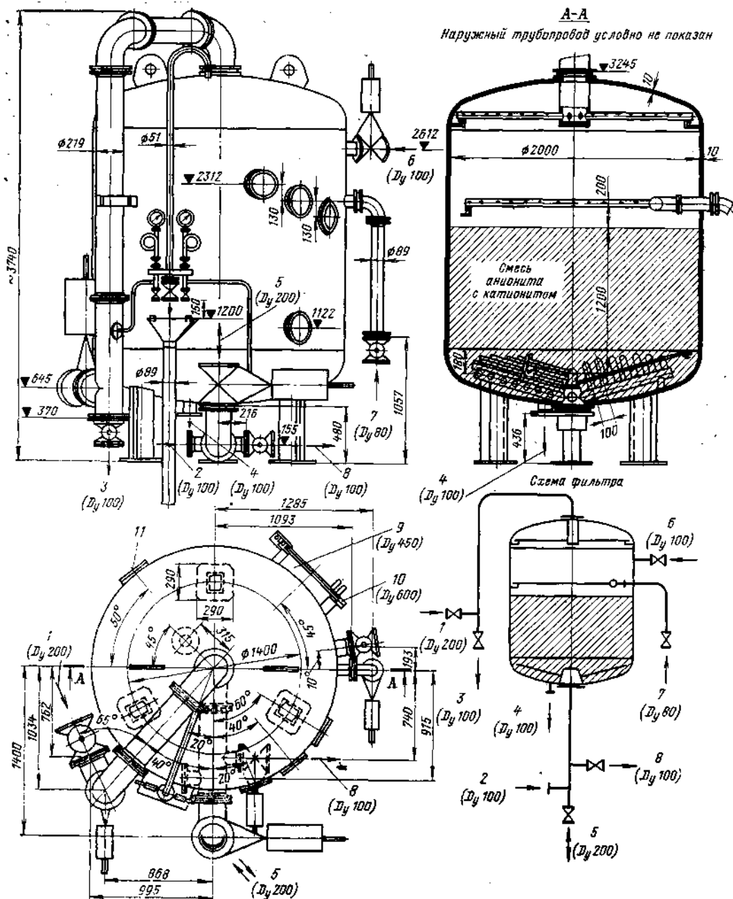
Рис. 7-21. Фильтр смешанного действия (ФСД) диаметром 2000 мм (с выносной регенерацией), ТКЗ.
