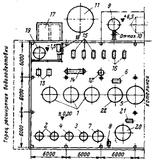
Рис. 9-6. Компоновка водоподготовительной установки по схеме рис. 9-5 с водород-катионитными фильтрами диаметром 2600 мм и натрий-катионитными фильтрами диаметром 1500 мм.
