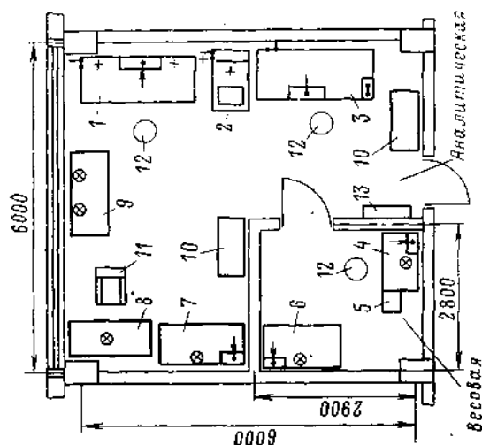
Рис. 12.3. Компонировка оборудования химической лаборатории типа II.
