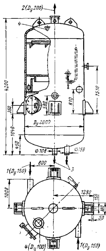
Рис. 7-43. Расширитель непрерывной продувки второй ступени СП-12 (ТКЗ). 1 — вход сепарируемой воды; 2 — выход отсепарированного пара; 3 — выход отсепарированной воды; 4 — штуцер для установки предохранительного клапана.
