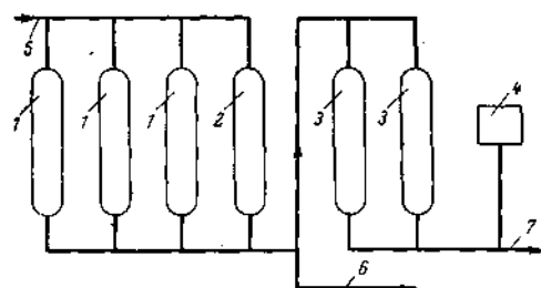
Рис. 9-3. Водоподготовительная установка для комбинированной котельной по схеме одноступенчатого натрий-катионирования для подпитки тепловой сети и двухступенчатого натрий-катионирования с нитратированием для паровых котлов.
