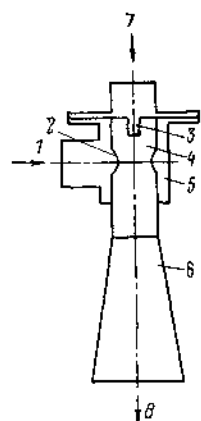
Рис. 13-9. Принципиальная схема водоструйного эжектора системы ЦКТИ.
