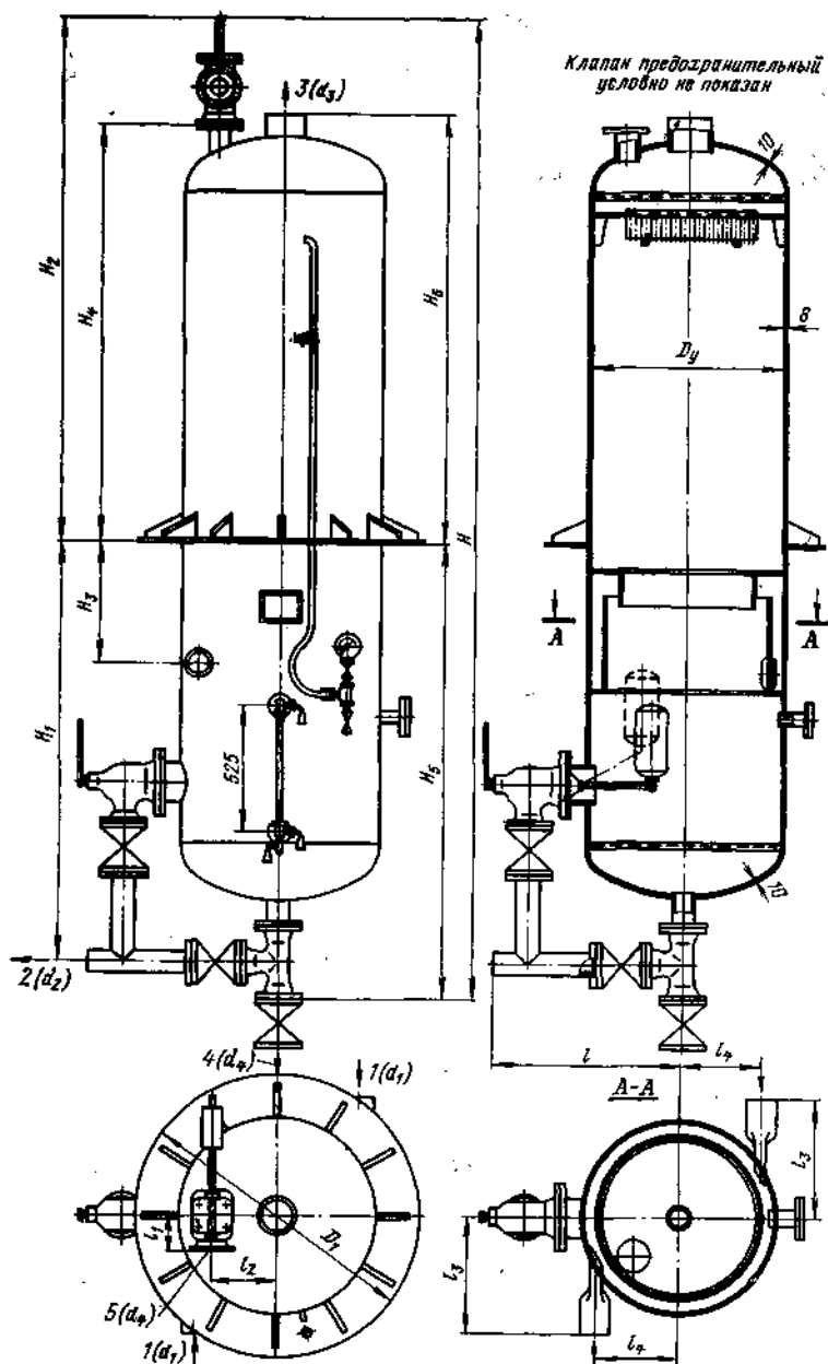
Рис. 7-41. Сепараторы непрерывной продувки СП-0,7 и СП-1,5 (ТКЗ), см. табл. 7-22. 1— вход продувочной воды; 2— выход отсепарированной воды; 3— выход отсепарированного пара; 4— пуск в дренаж; 5— предохранительный клапан.
