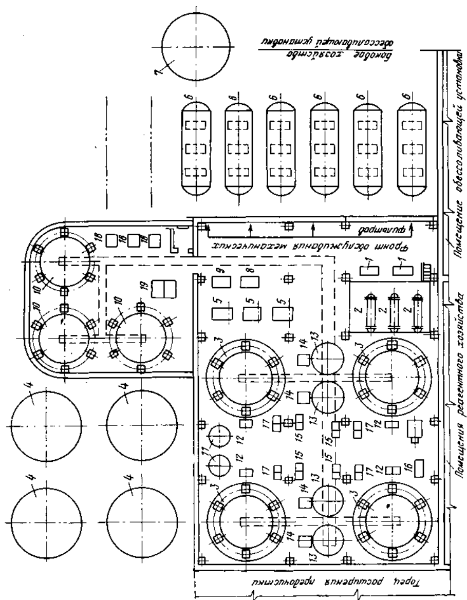
Рис. 9-9. Компонировка установок предварительной очистки (предочистки) поверхностной воды.
