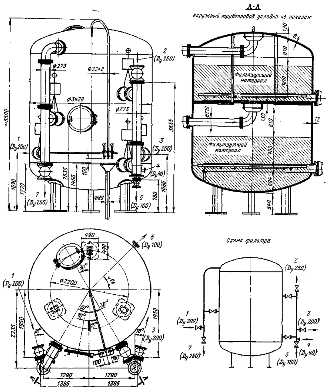
Рис. 7-4. Фильтр осветлительный двухкамерный диаметром 3400 мм (ТКЗ).
