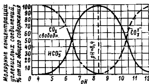
Рис. 10-4. График соотношений \text{CO}_2 , \text{HCO}_3^- и \text{CO}_3^{2-} в зависимости от pH воды.
