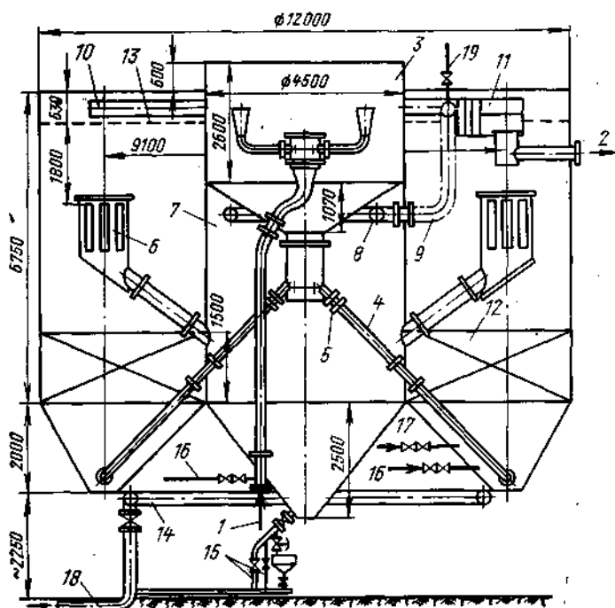
Рис. 8-7. Осветлитель для коагуляции (проект Хо ТЭП—ВТИ) производительностью 350 м 3 /ч.
