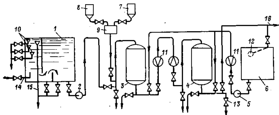
Рис. 2-14. Принципиальная схема очистки конденсата от масла (нефтепродуктов). 1 — бак-отстойник конденсата; 2 — насос загрязненного (отстоявшегося) конденсата; 3 — механический фильтр; 4 — фильтр активированного угля (ФАУ); 5 — насос для промывки фильтров; 6 — бак для промывки хлопьев гидрооксида алюминия; 7 — мерник раствора коагулянта; 8 — мерник раствора щелочи; 9 — бак для получения хлопьев гидрооксида алюминия; 10 — пробоотборное устройство; 11 — расходомер показывающий; 12 — автоматический запорный клапан; 13 — отбор пробы очищенного конденсата; 14 — подвод загрязненного конденсата на очистку; 15 — сброс в дренаж; 16 — очищенный конденсат в деаэратор.
