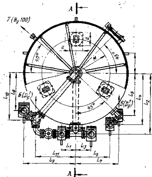
Рис. 7-19. Фильтры ионообменные противоточные водород-катионитные с «зажатым слоем» диаметром от 2000 до 3400 мм (ТКЗ), см. табл. 7-13.
