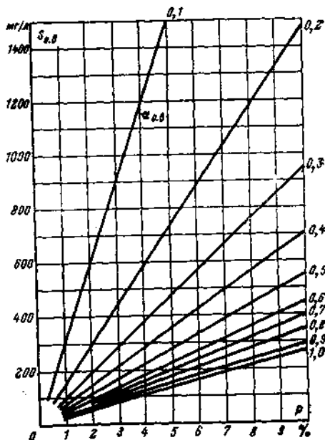
Рис. 4-5. Определение величины продувки котлов, %, в зависимости от сухого остатка обработанной воды S_{0.в} при S_{к.в} = 3000 мг/л.
