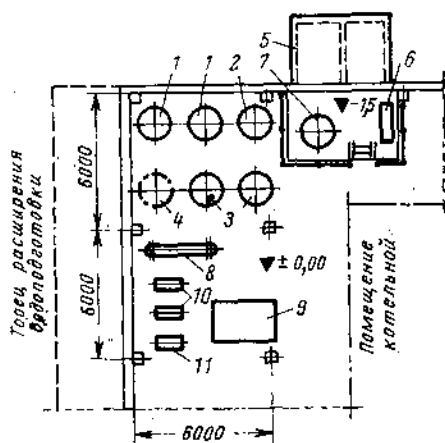
Рис. 9-8. Компоновка водоподогревательной установки по схеме рис. 9-7 с фильтрами диаметром 1000 мм.
