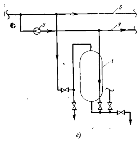
Рис. 6-9. Схема взрыхляющей промывки фильтров.
