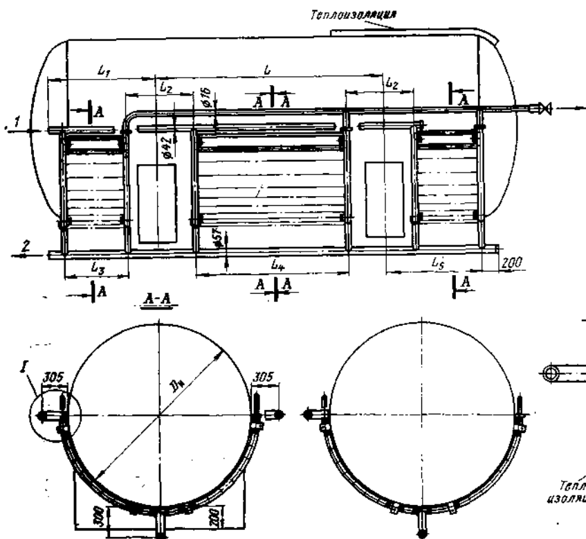
Рис. 7-60. Подогреватели к бакам для хранения кислоты и щелочи (ТКЗ).
