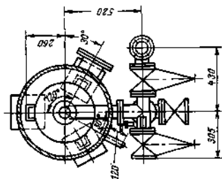
Рис. 7-57. Содержатель реактивов D_y = 600 мм (СЗТМ). 1 — вход воды для растворения соли; 2 — вход промывочной воды; 3 — выход раствора соли; 4 — дренаж; 5 — фильтрующий материал.
