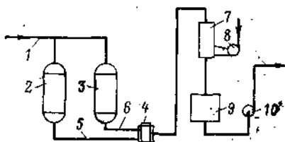
Рис. 2-9. Схема параллельного водород-натрий-катионирования.
