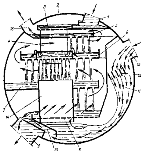
Рис. 13-7. Принципиальная схема двухступенчатого вакуумного деаэратора ЦКТИ — производительностью 400—3200 т/ч.
