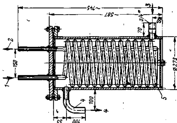
Рис. 7-45. Охладитель отбора проб пара и воды ЗН-249-67 (СЭТМ).
